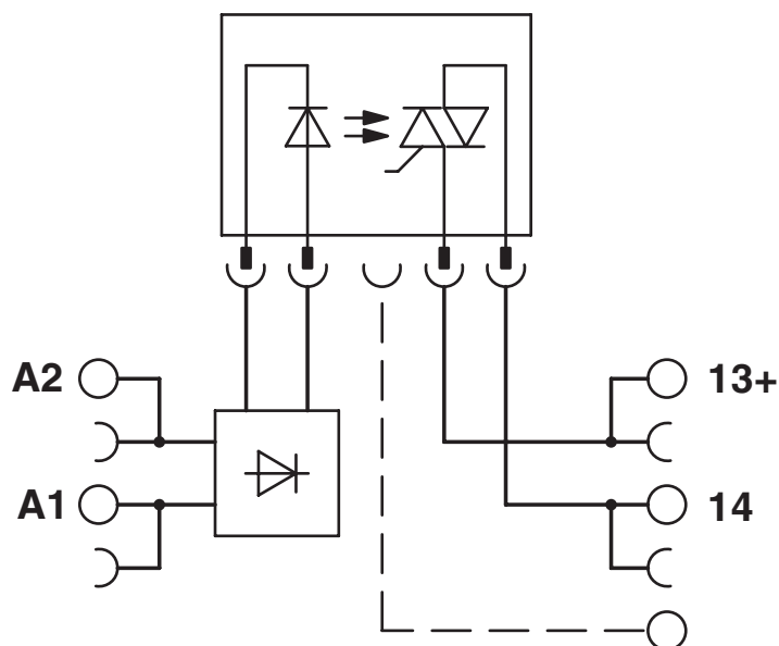
Schemat
