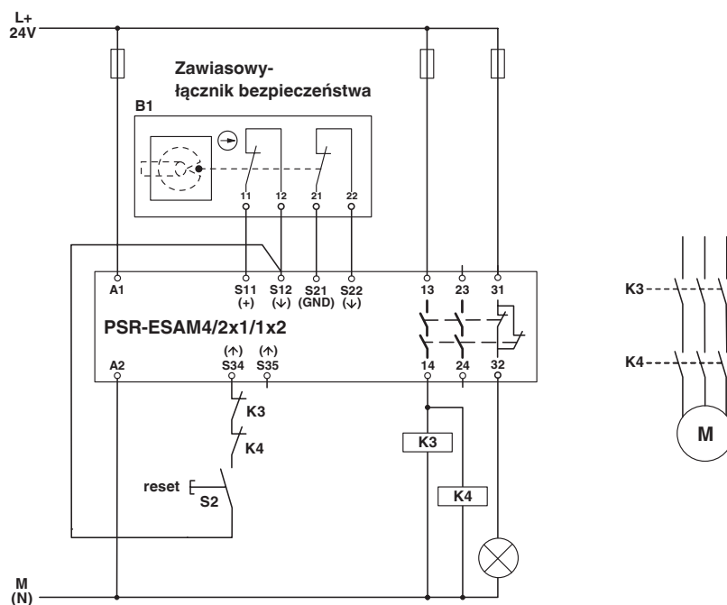
Schemat
