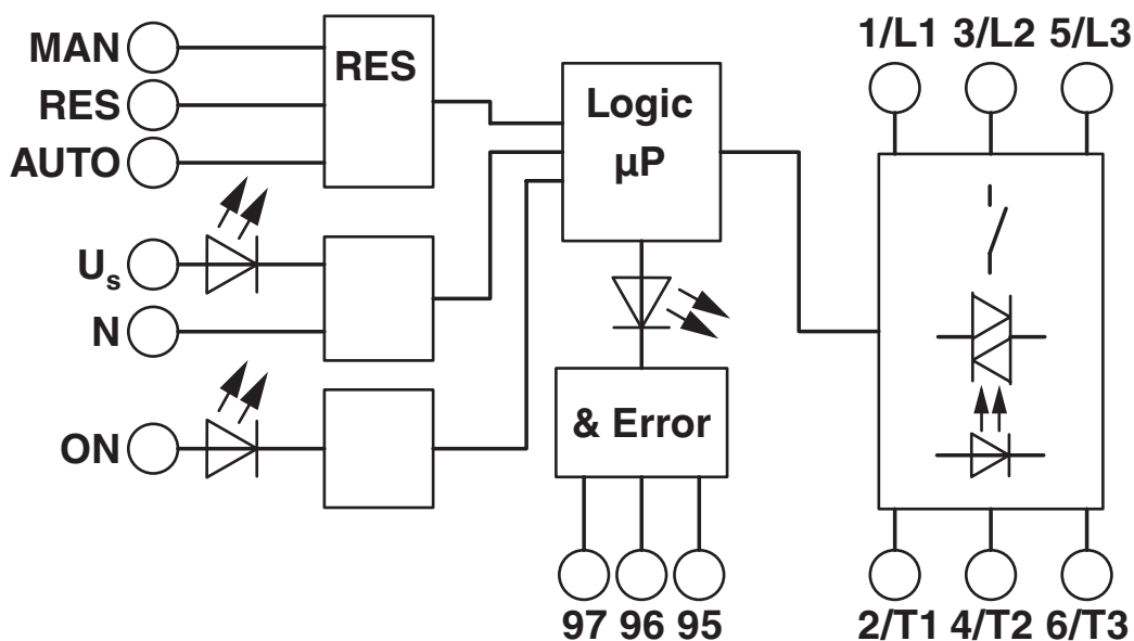
Schemat blokowy
