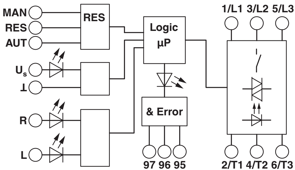
Schemat blokowy
