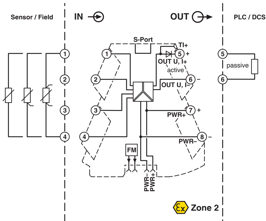
Schemat blokowy
