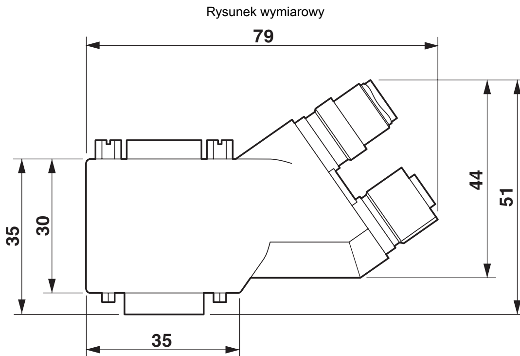
Rysunek wymiarowy SUBCON-PLUS..35...M12, wersja 35°
