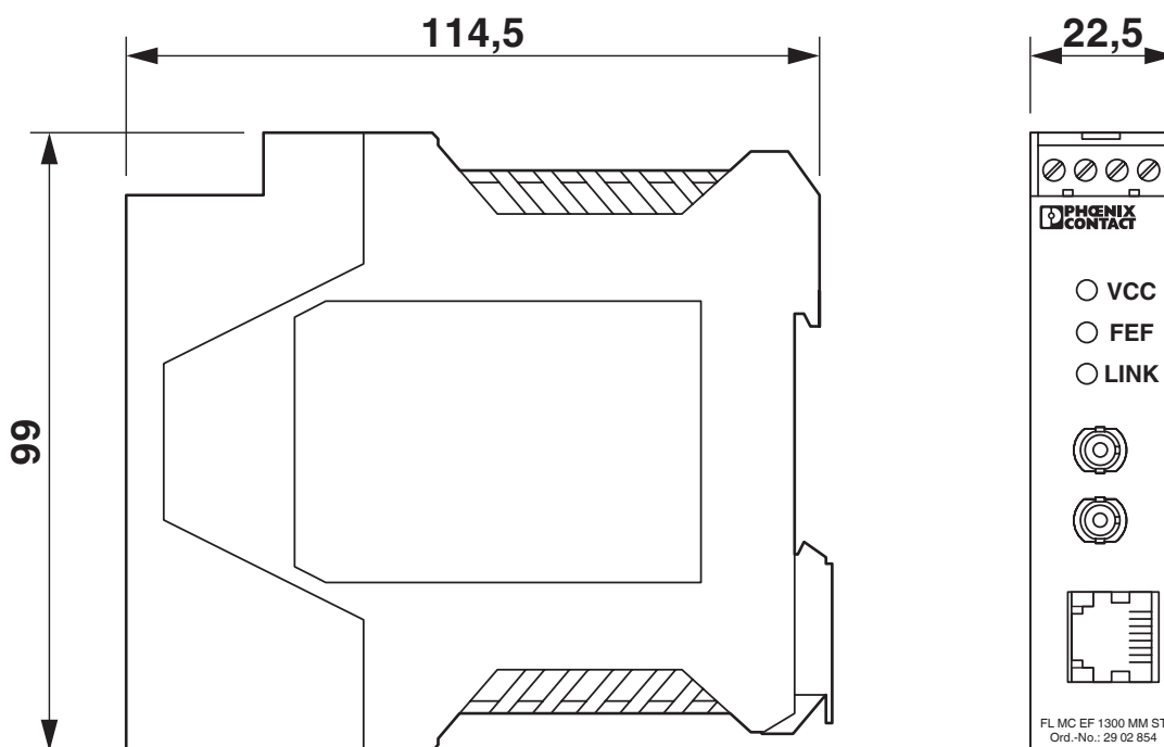
Rysunek wymiarowy
