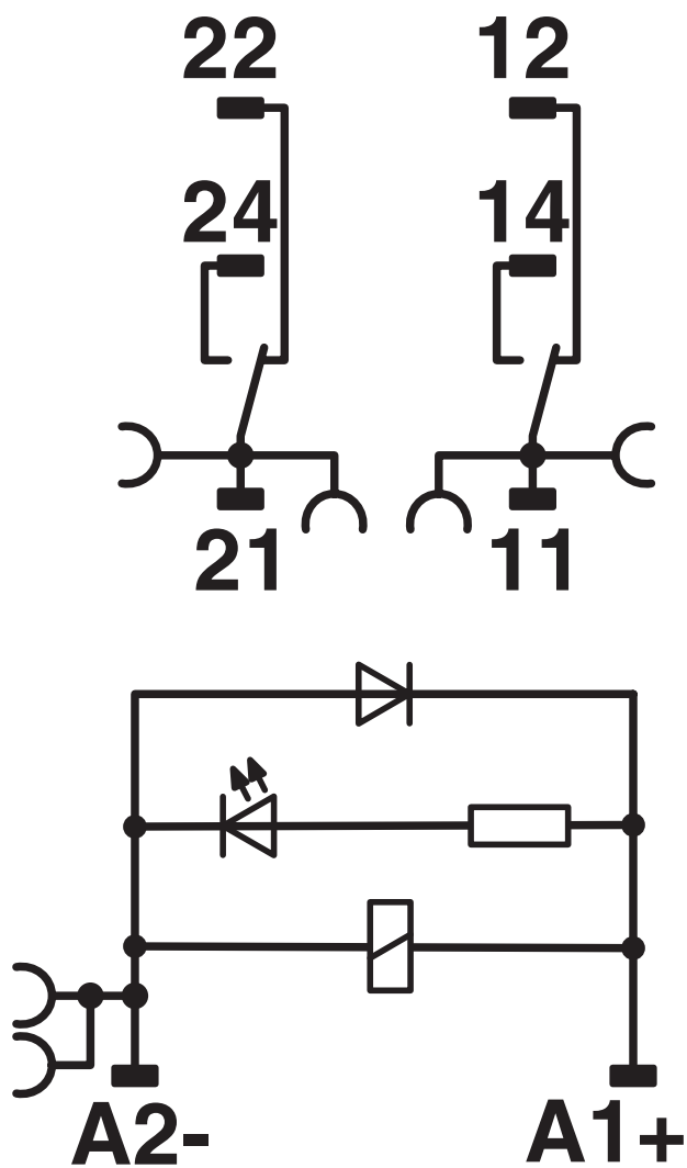
Schemat
