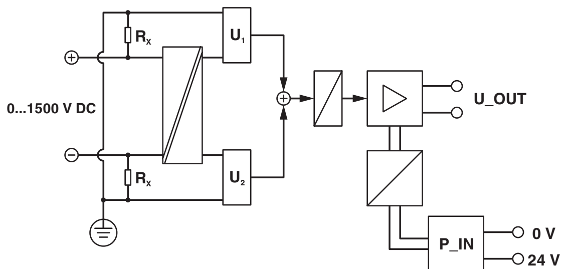
Schemat blokowy
