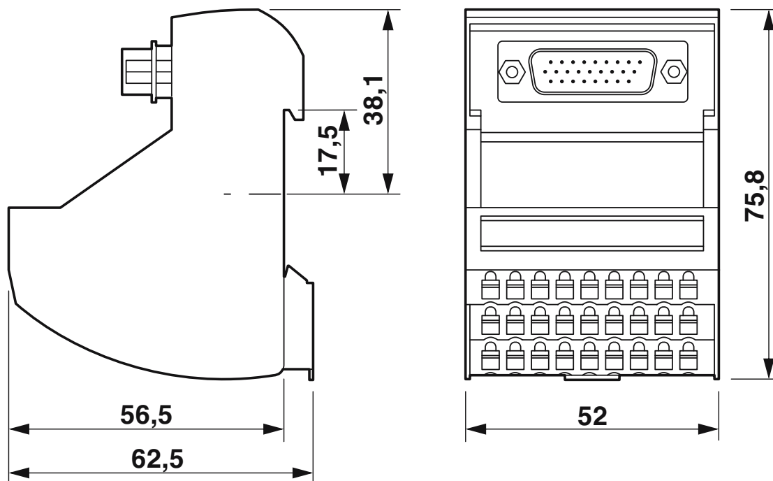
Rysunek wymiarowy
