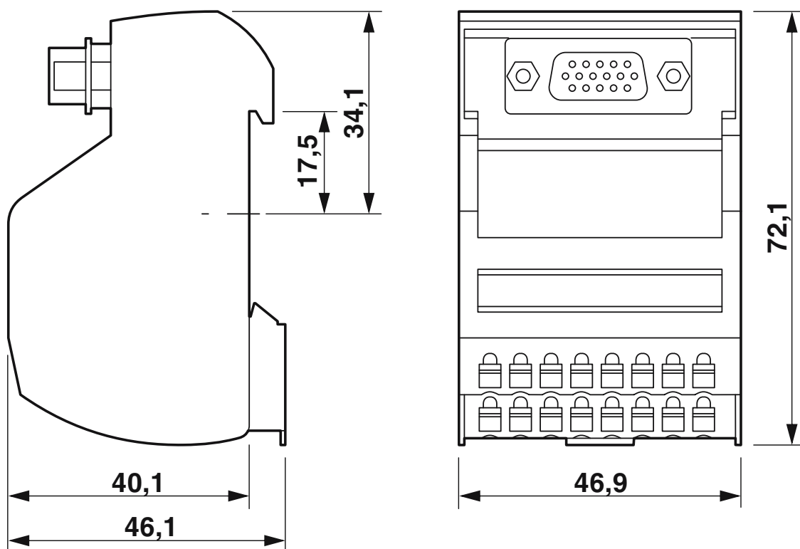
Rysunek wymiarowy
