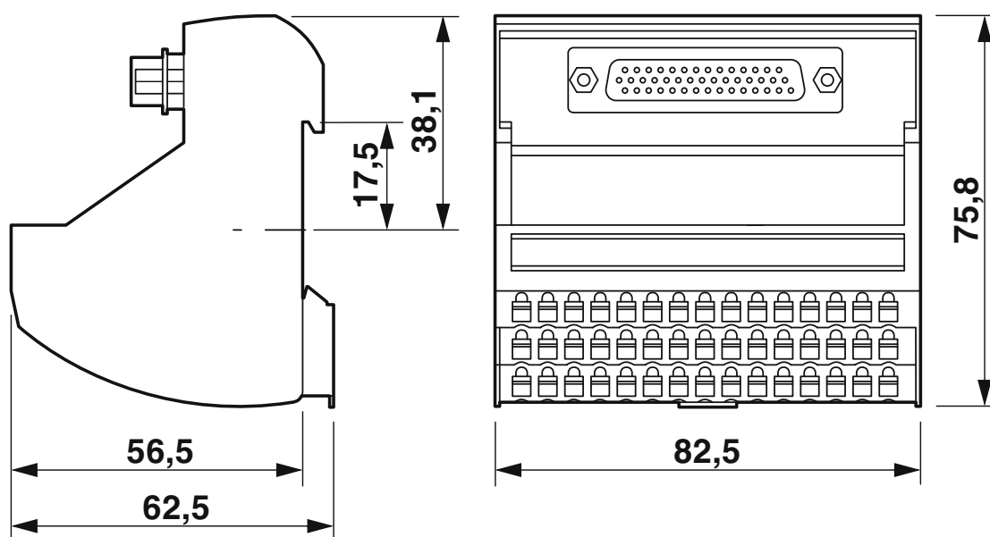
Rysunek wymiarowy
