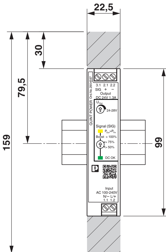
Rysunek wymiarowy
