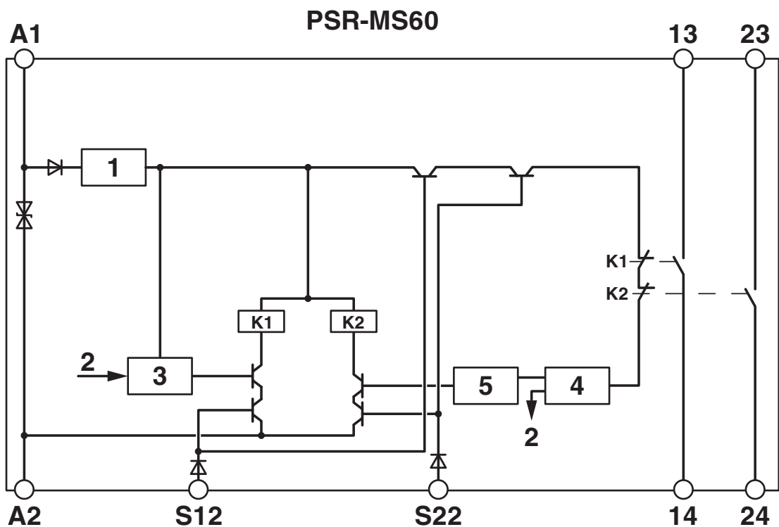
Schemat blokowy
