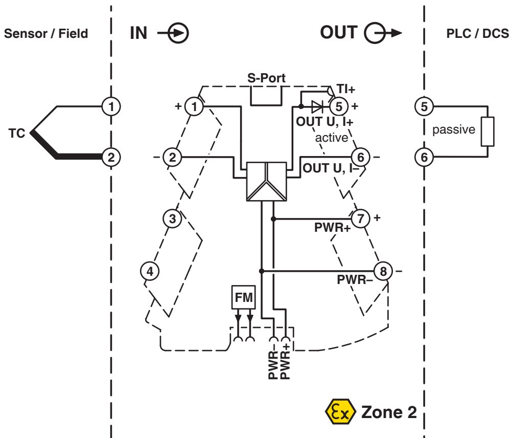
Schemat blokowy
