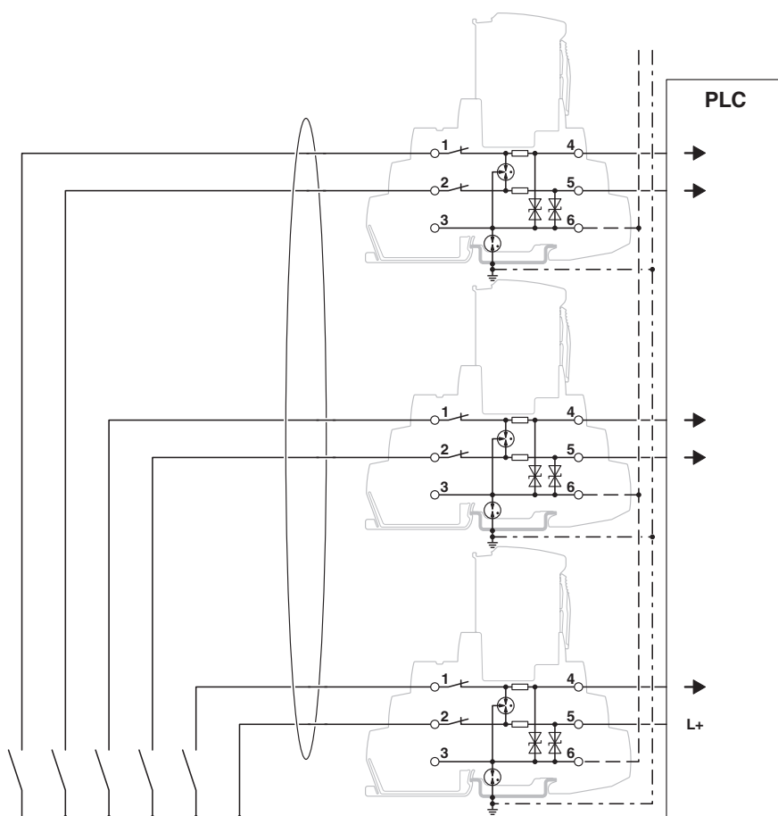
rysunek aplikacji
