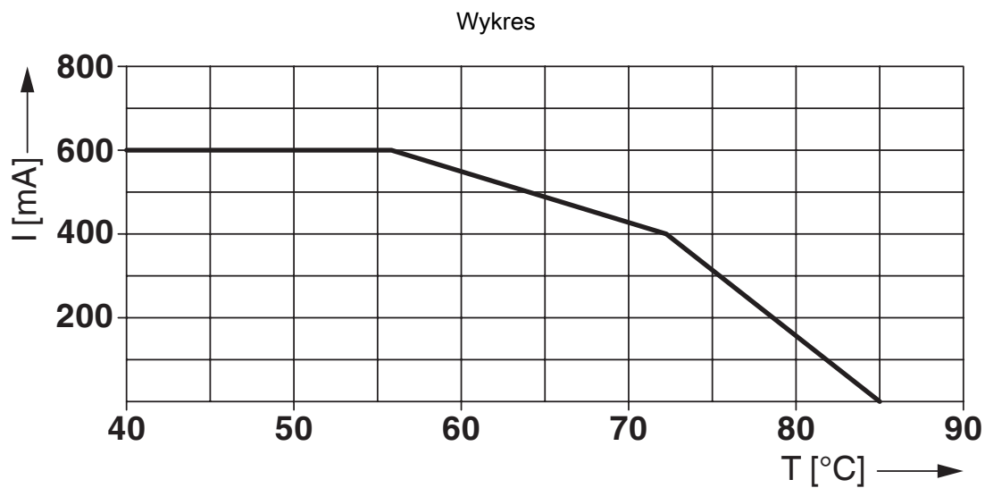
Wykres obniżenia parametrów znamionowych przy 30 V AC
