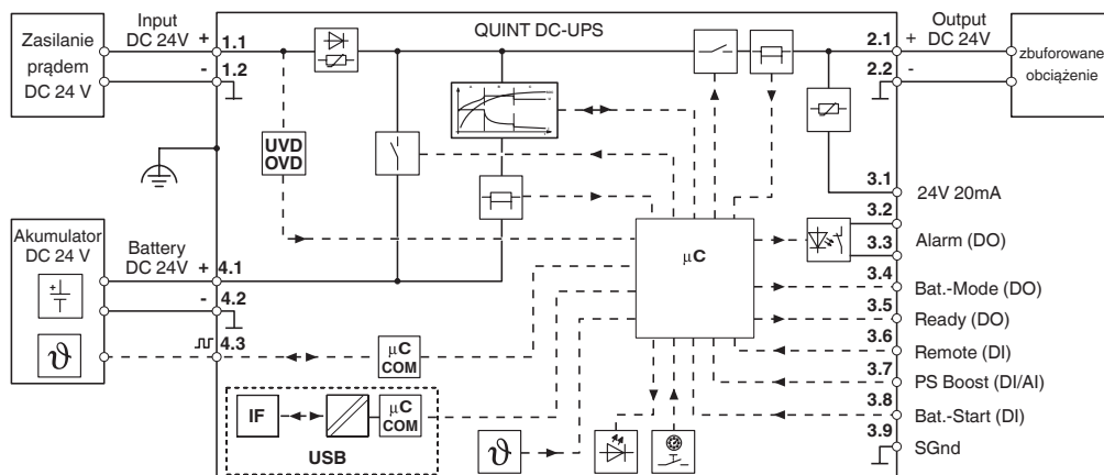
Schemat blokowy
