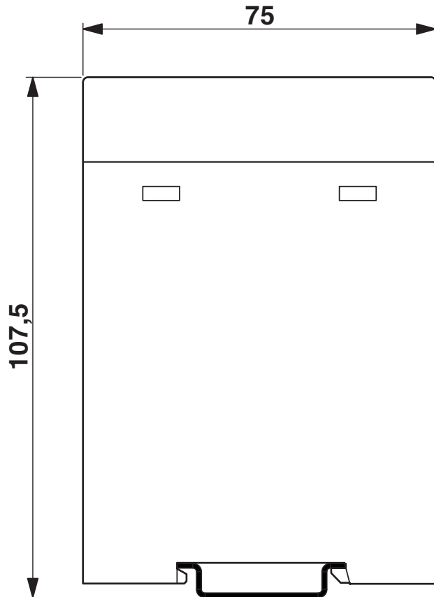
Rysunek wymiarowy
