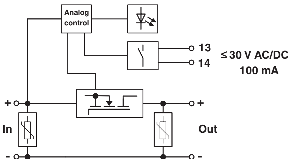
Schemat blokowy
