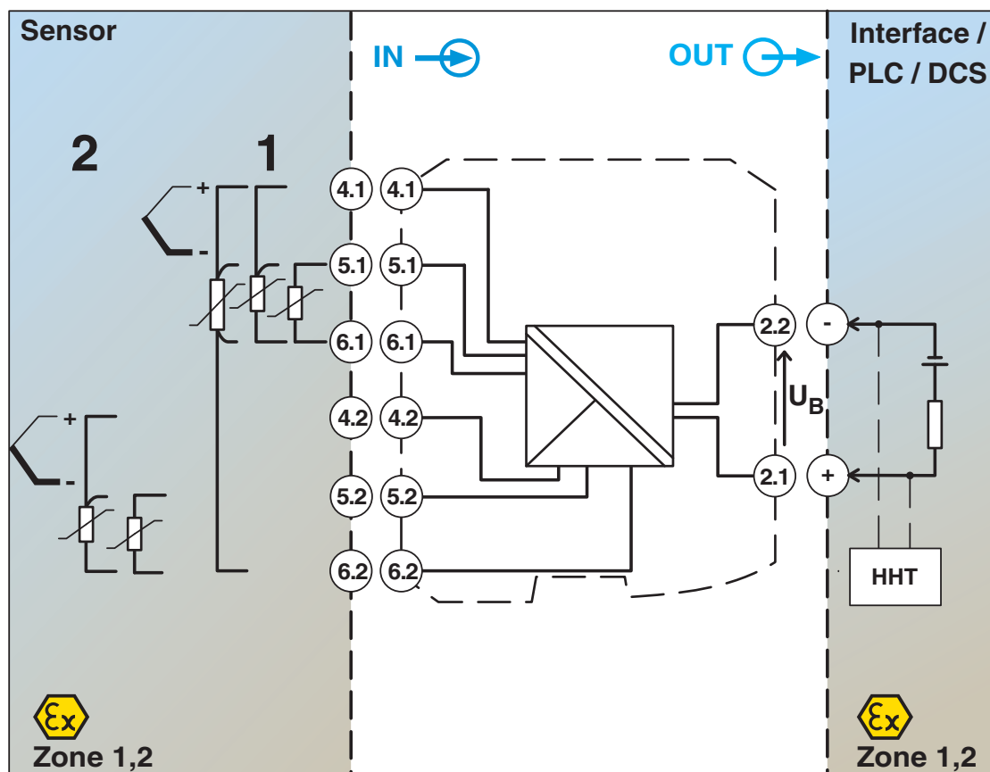
Schemat blokowy MACX MCR-EX-TS-I-OLP
