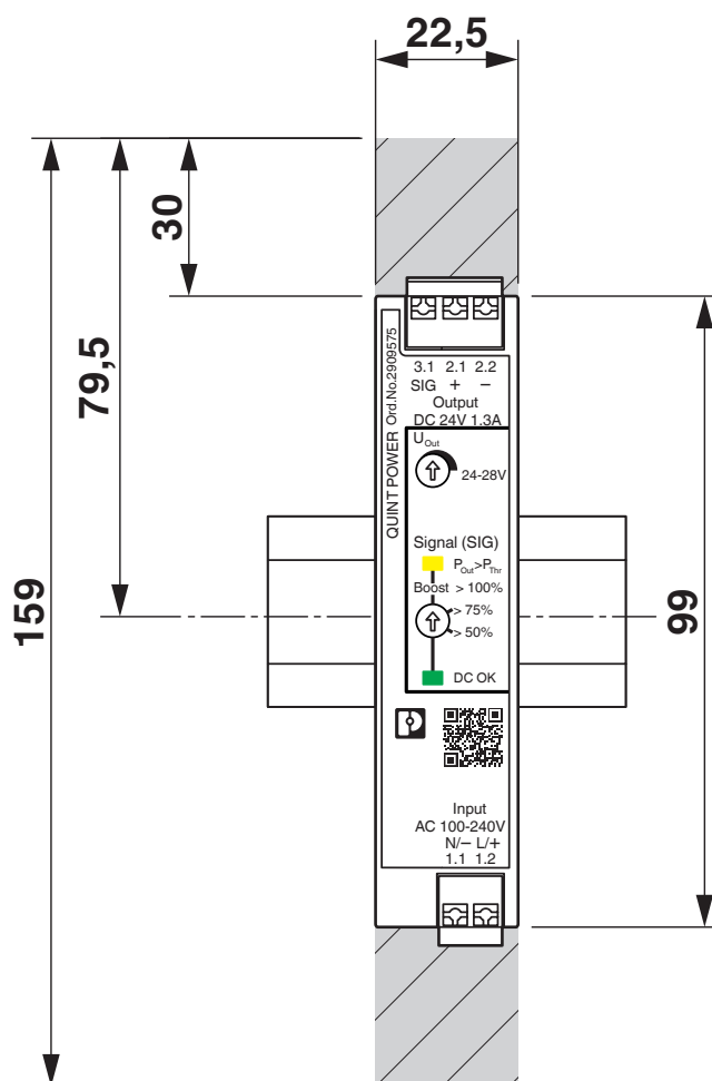
Rysunek wymiarowy
