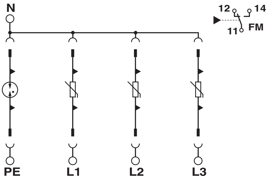
Schemat
