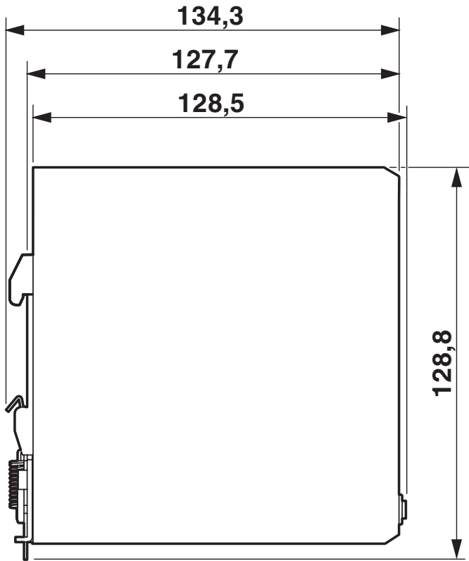
Rysunek wymiarowy
