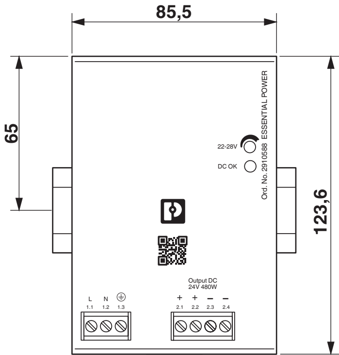
Rysunek wymiarowy
