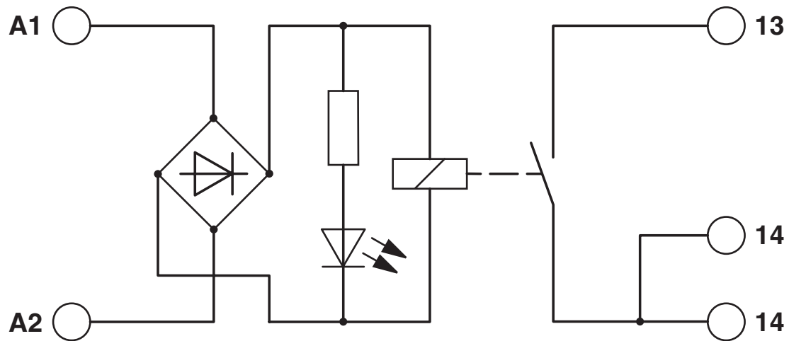
Schemat
