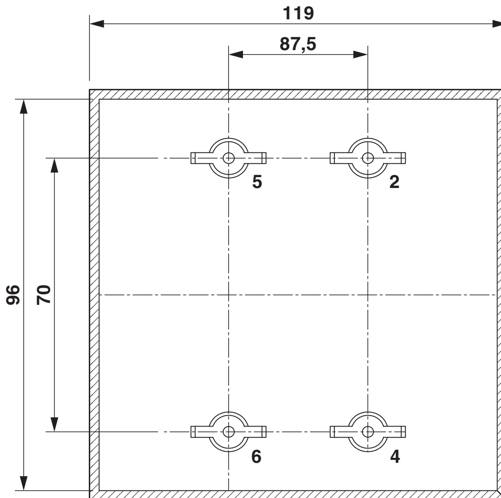
Rysunek wymiarowy
