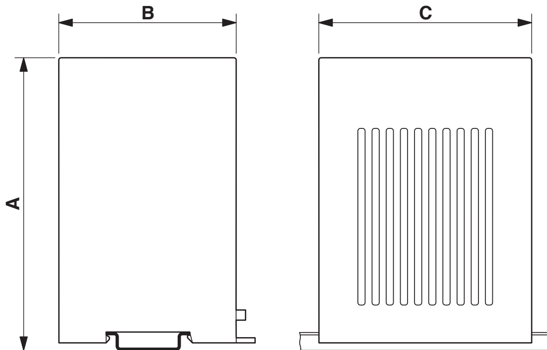
Rysunek wymiarowy
