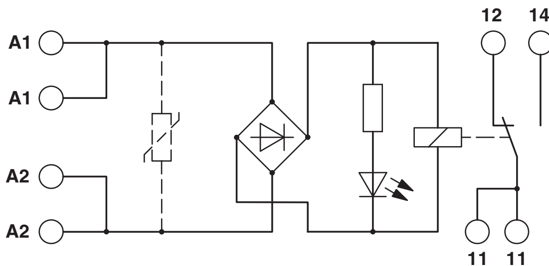
Schemat
