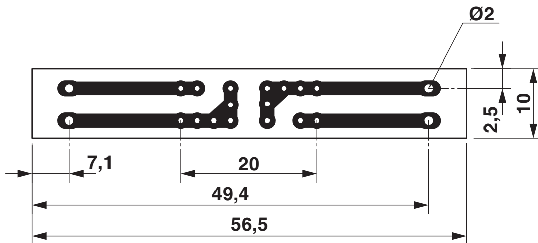
Rysunek wymiarowy
