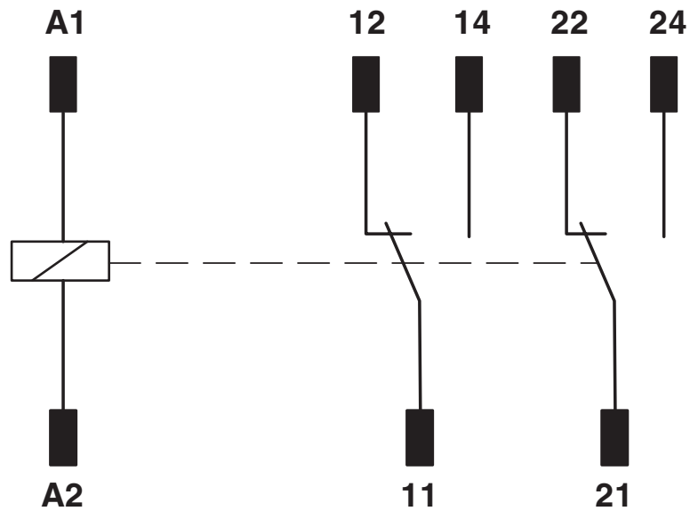
Schemat blokowy
