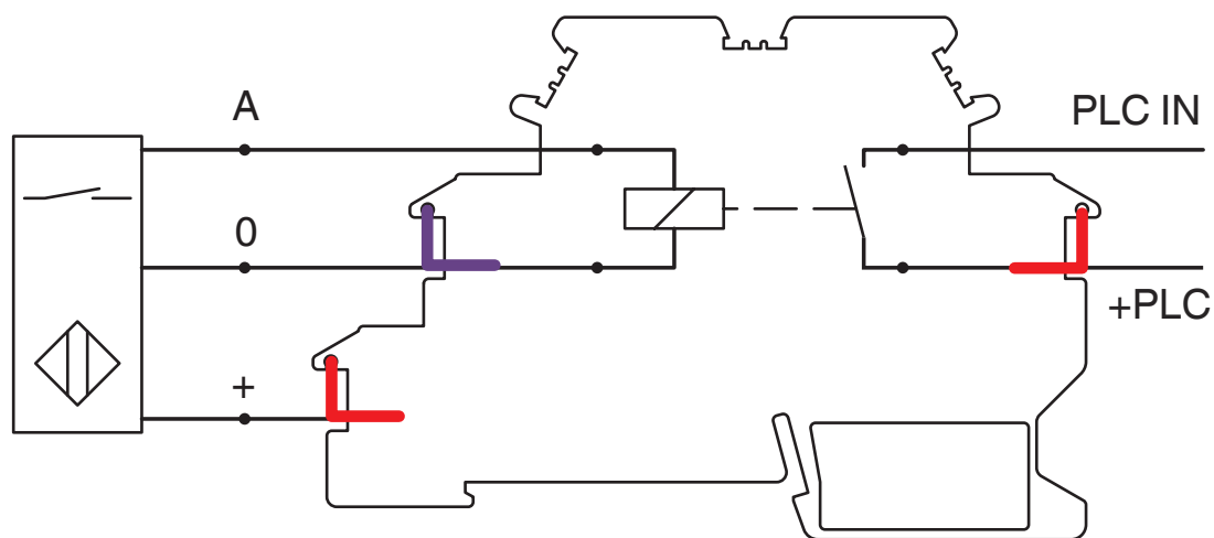
Przyporządkowanie przyłączy DEK-REL-...SEN
