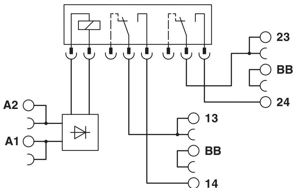
Schemat
