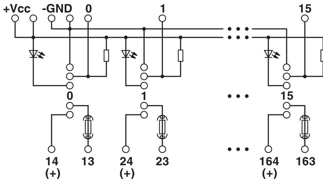
Schemat
