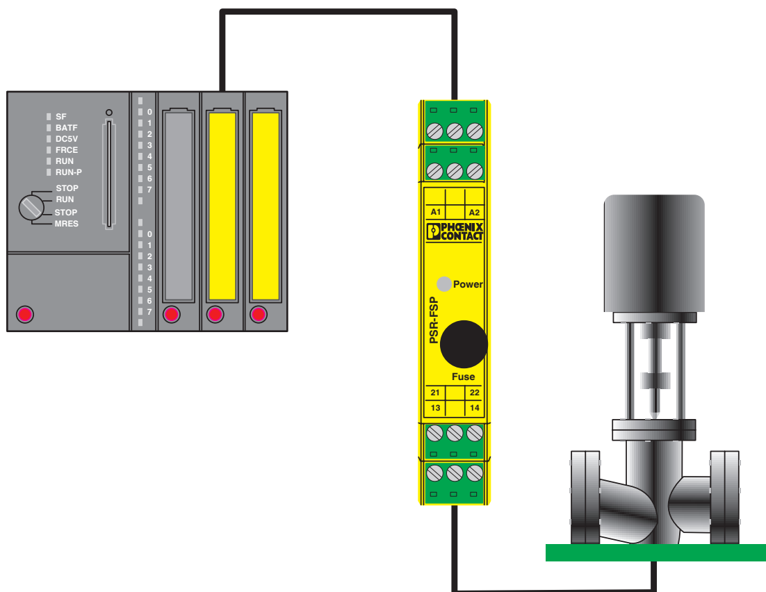
rysunek aplikacji
