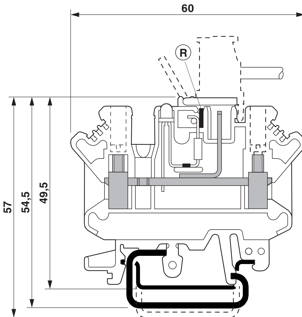
Rysunek wymiarowy
