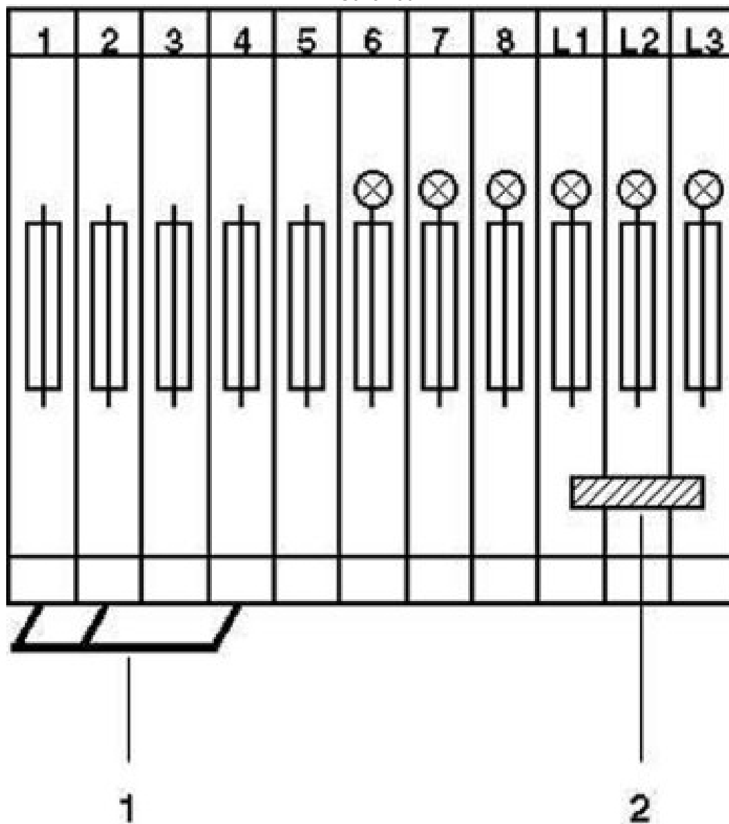
Schemat
