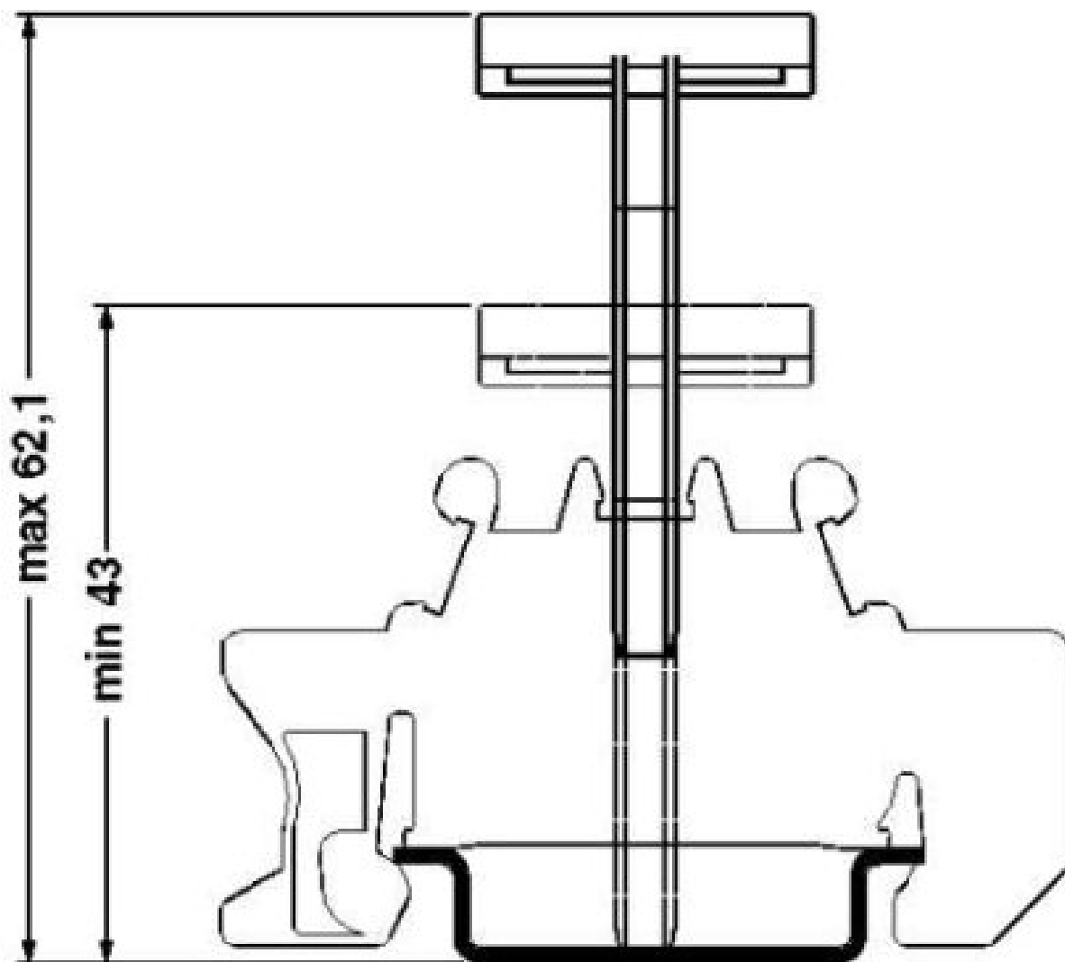
Rysunek wymiarowy
