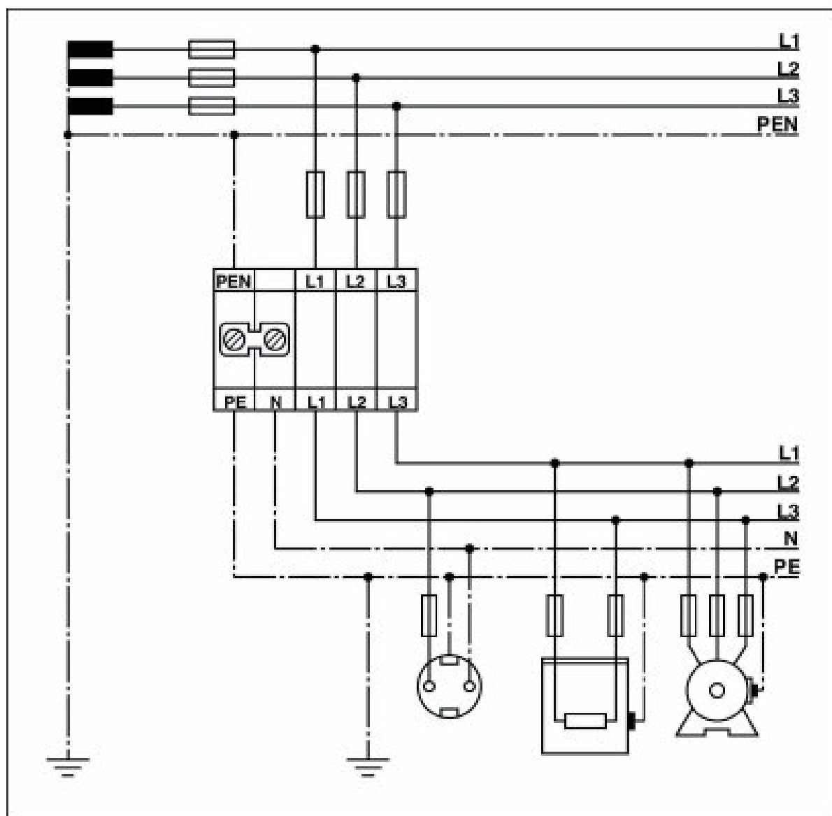
rysunek złączy
