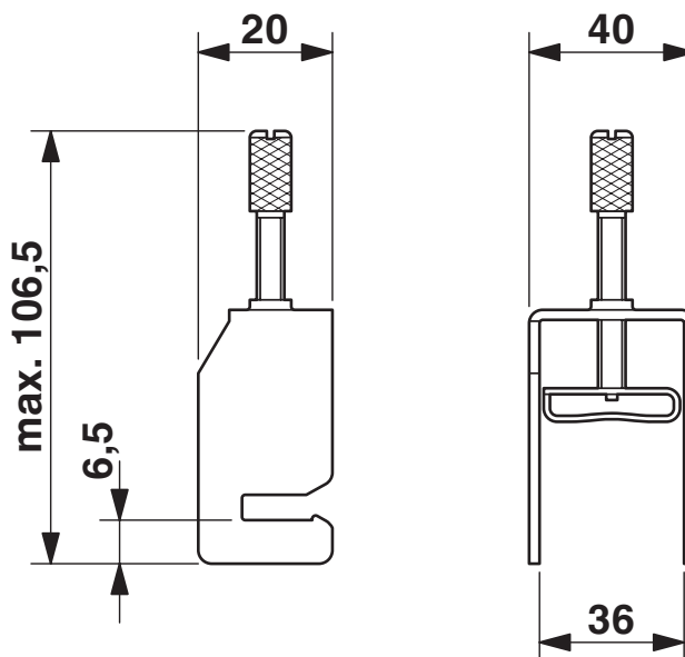
Rysunek wymiarowy
