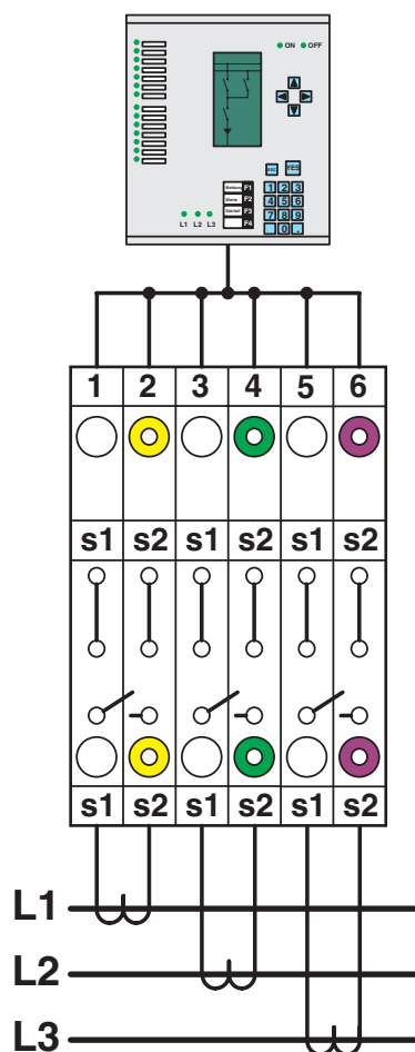
Rysunek schematyczny
