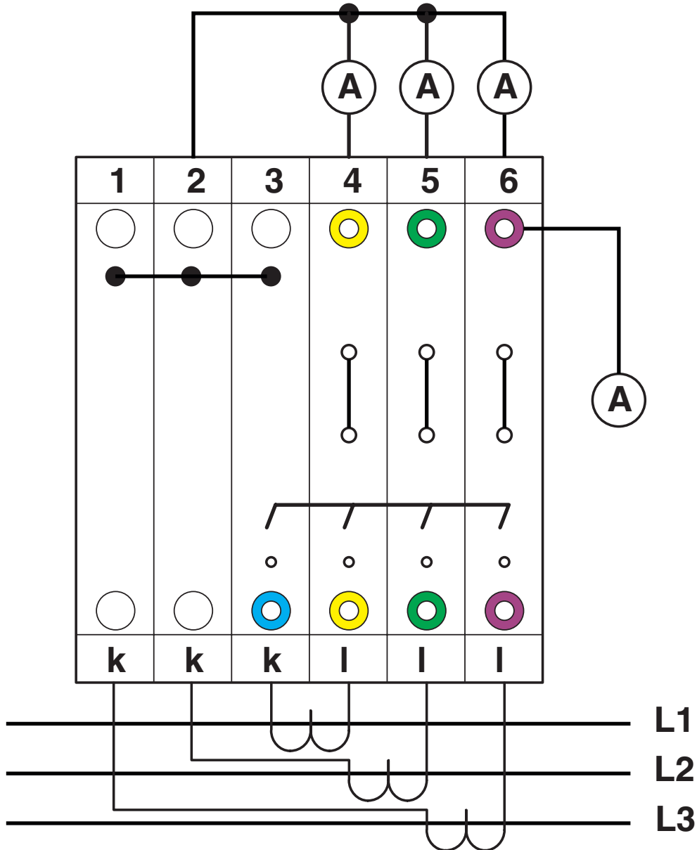
rysunek złączy
