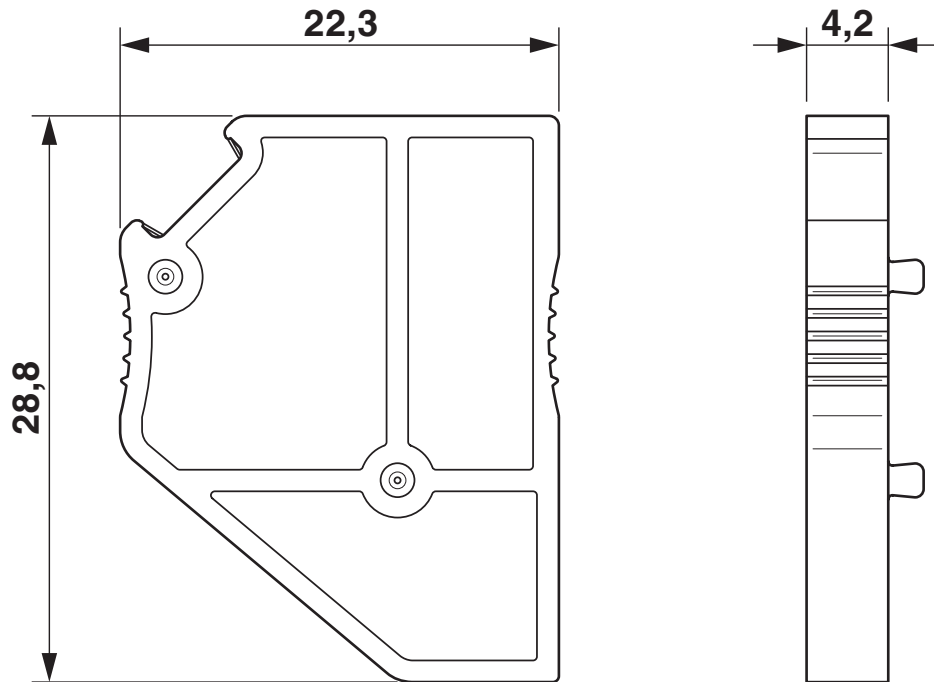
Rysunek wymiarowy
