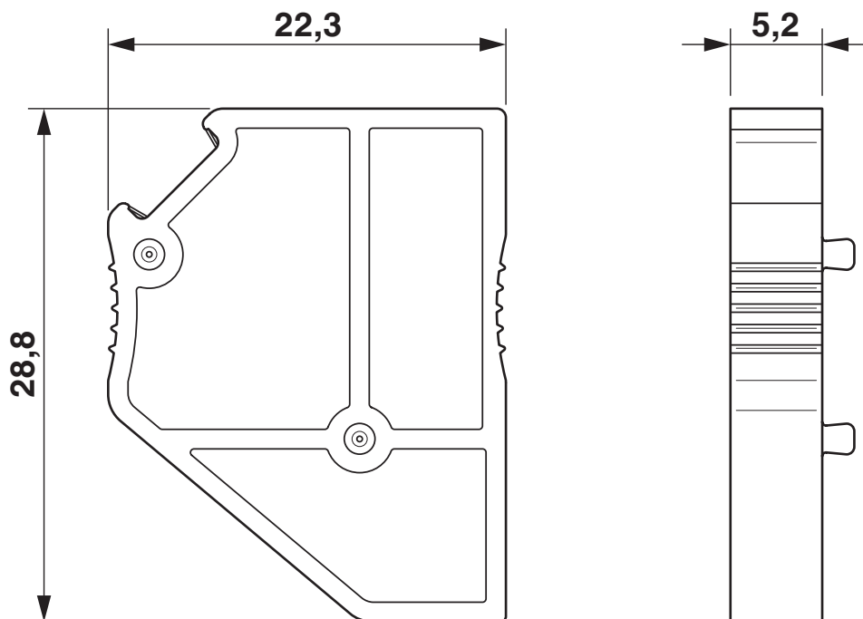
Rysunek wymiarowy
