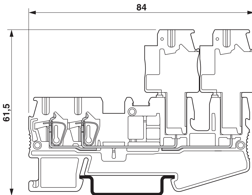
Rysunek wymiarowy
