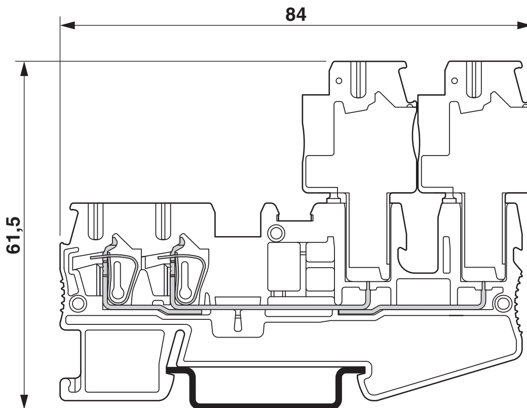
Rysunek wymiarowy
