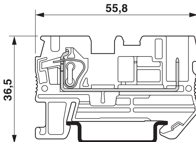
Rysunek wymiarowy
