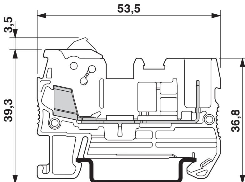
Rysunek wymiarowy
