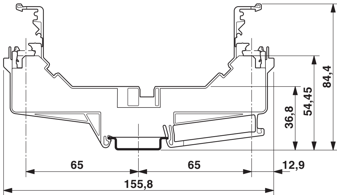
Rysunek wymiarowy
