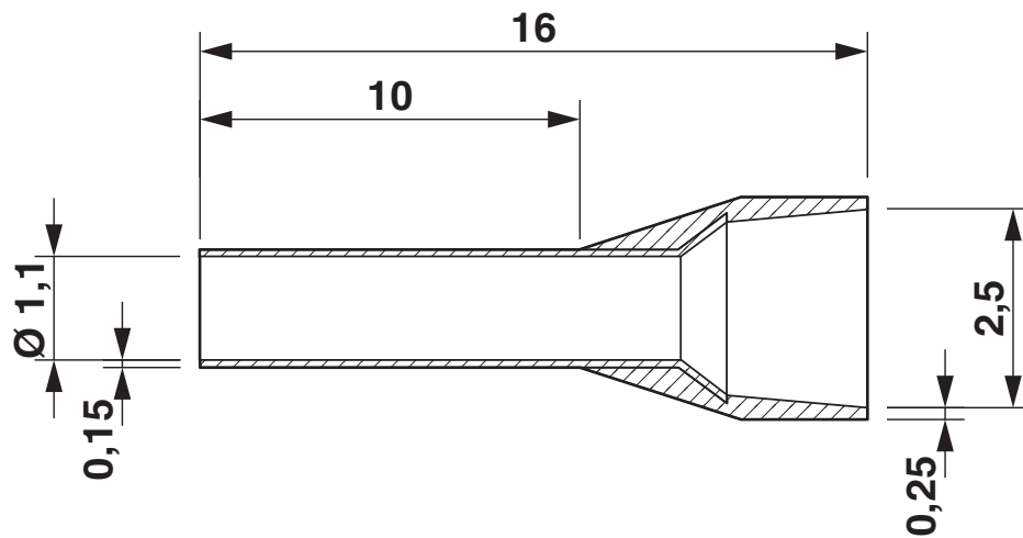
Rysunek wymiarowy
