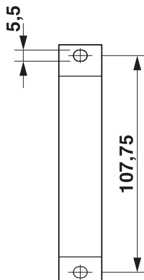
Rysunek wymiarowy
