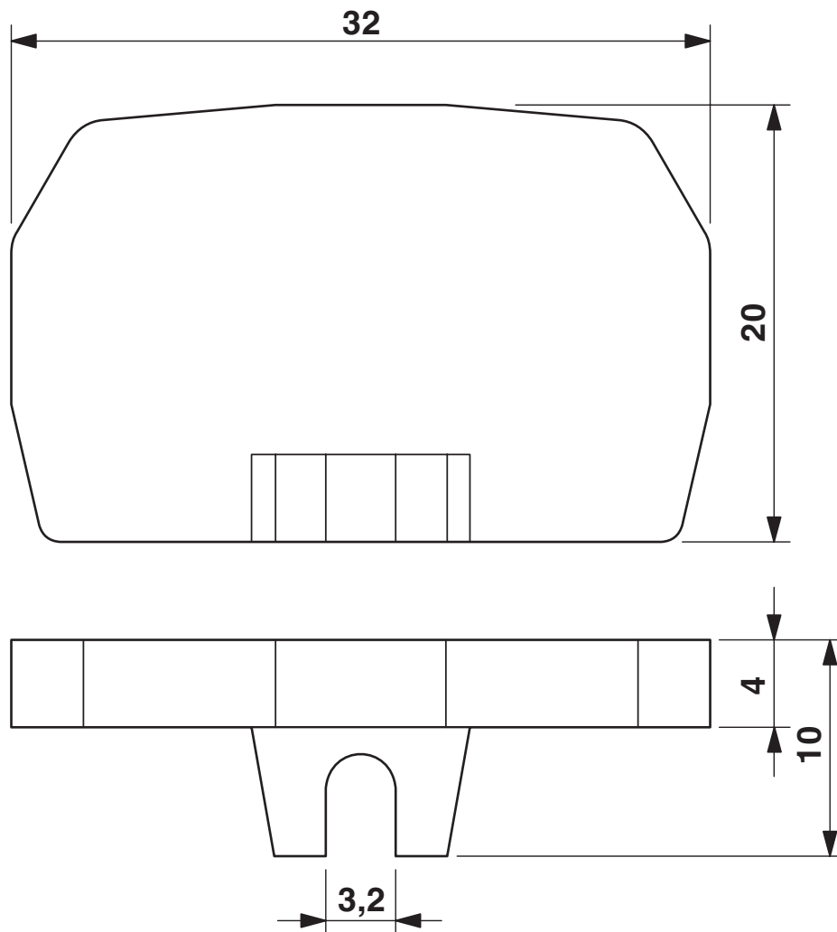
Rysunek wymiarowy
